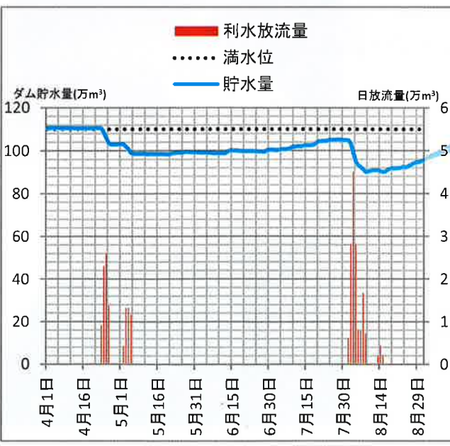
● 後谷ダム (有効貯水量110万 m^3 ) 計画受益面積880ha(現供給面積440ha)
